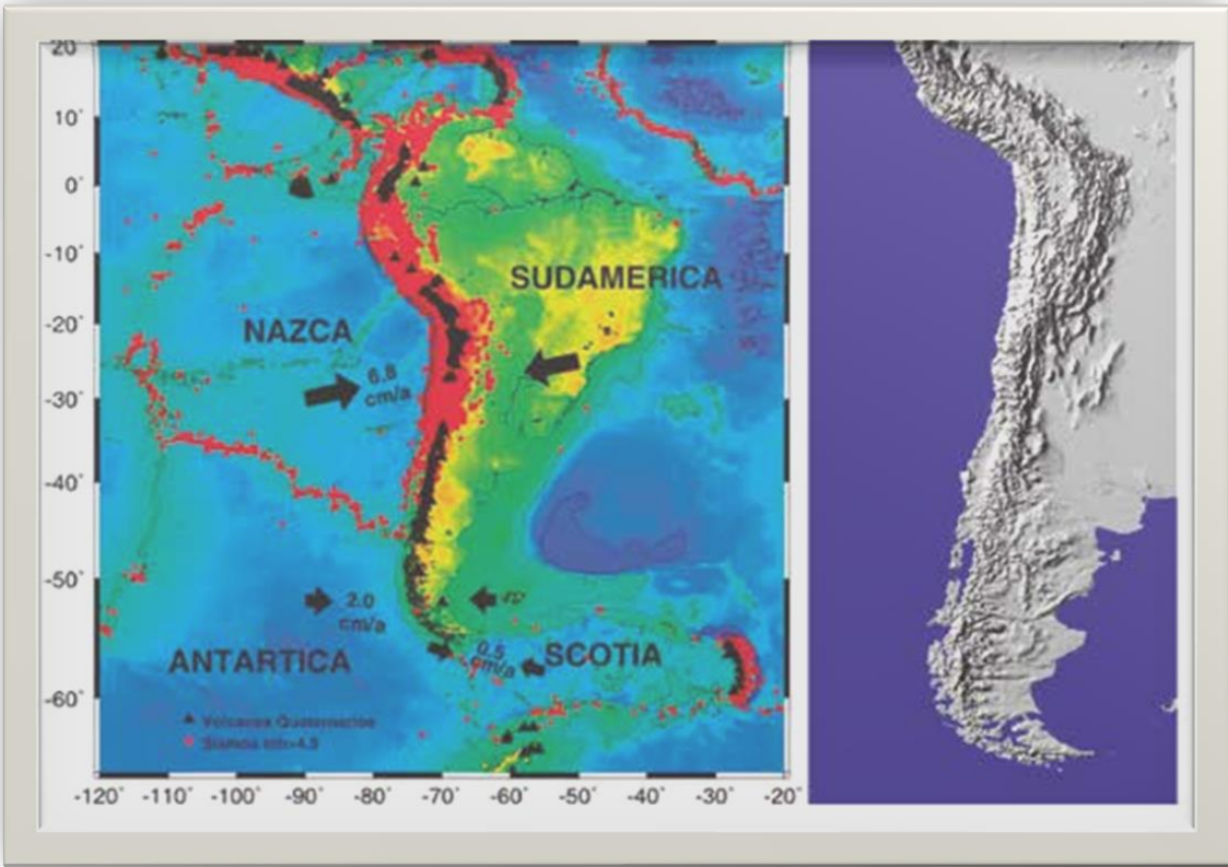
Figura N°14: Marco Tectónico de Chile
