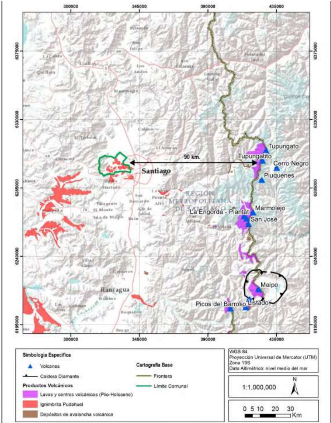
Mapa N°20. Mapa de ubicación de volcanes cercano de la comuna de Pudahuel
