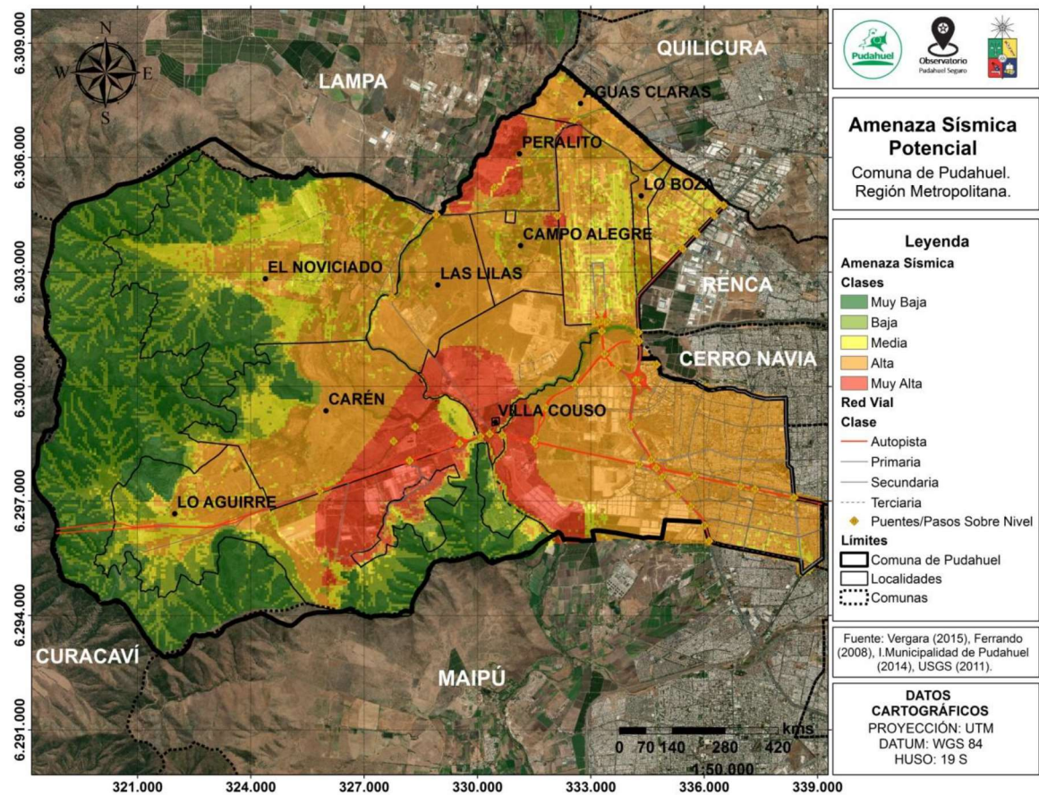
Mapa N°8. Amenaza Sísmica Potencial en la Comuna de Pudahuel
