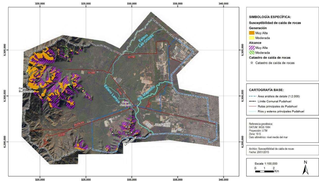
Mapa N°16. Susceptibilidad de caída de rocas.
