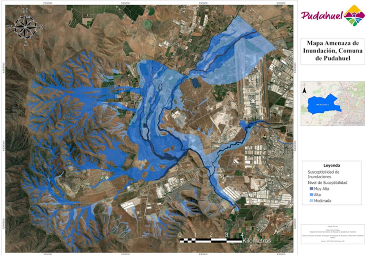
Mapa N°11. Mapa de amenaza de inundación en la comuna de Pudahuel.
