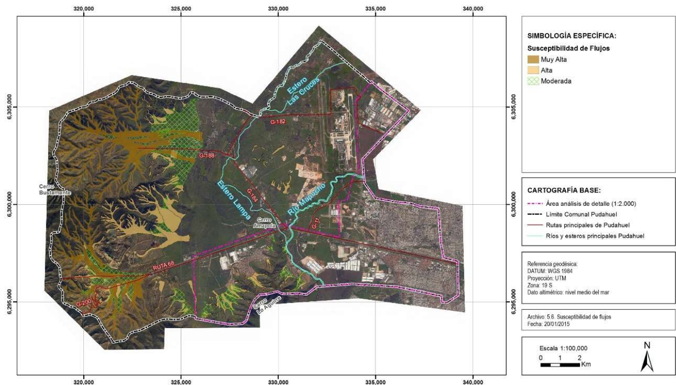
Mapa N°19. Susceptibilidad de flujos de barro y/o detritos.
