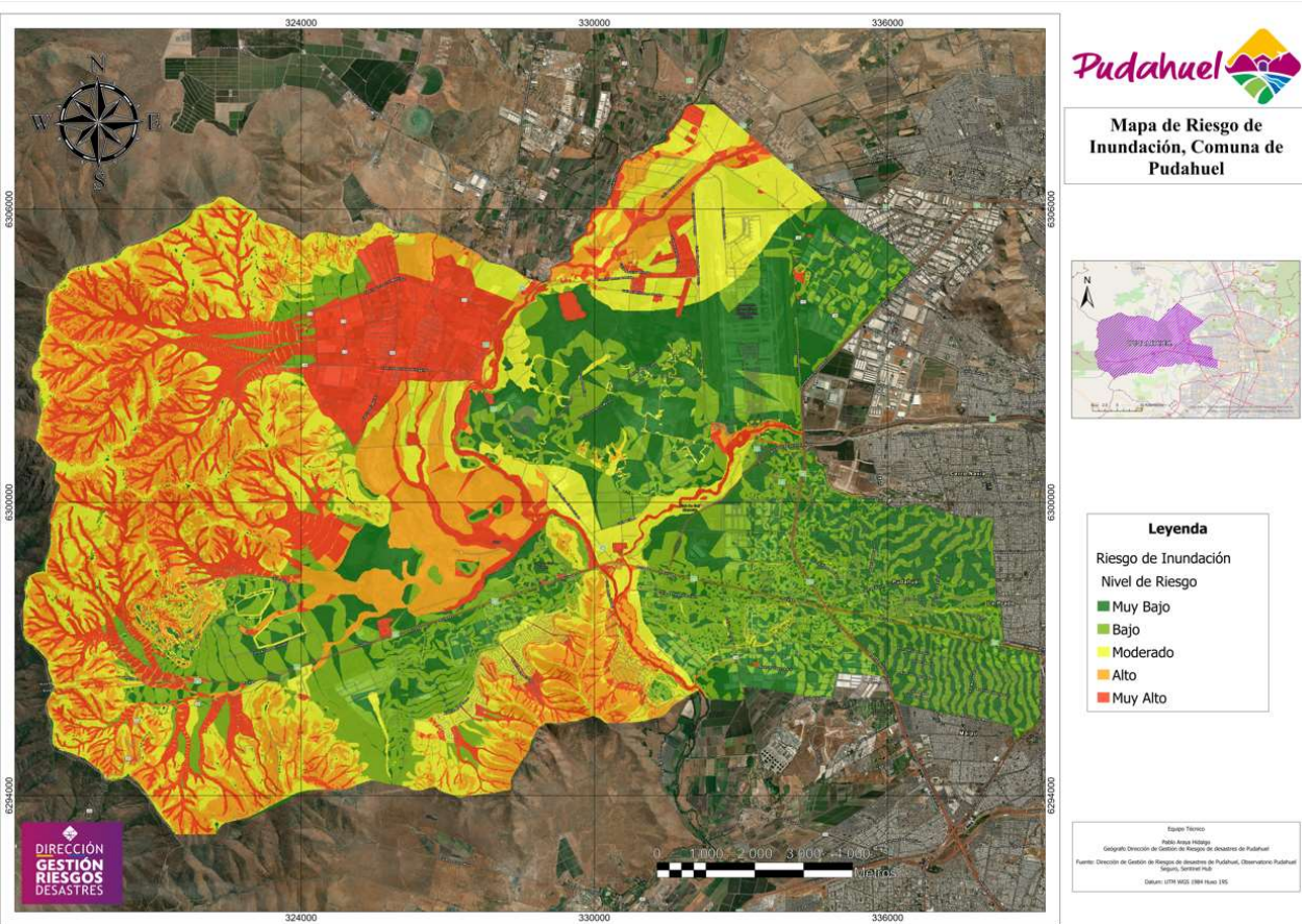
Mapa N° 14. Mapa de riesgo de inundaciones de la comuna de Pudahuel.
