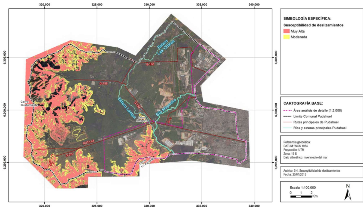
Mapa N°17. Susceptibilidad de deslizamientos.
