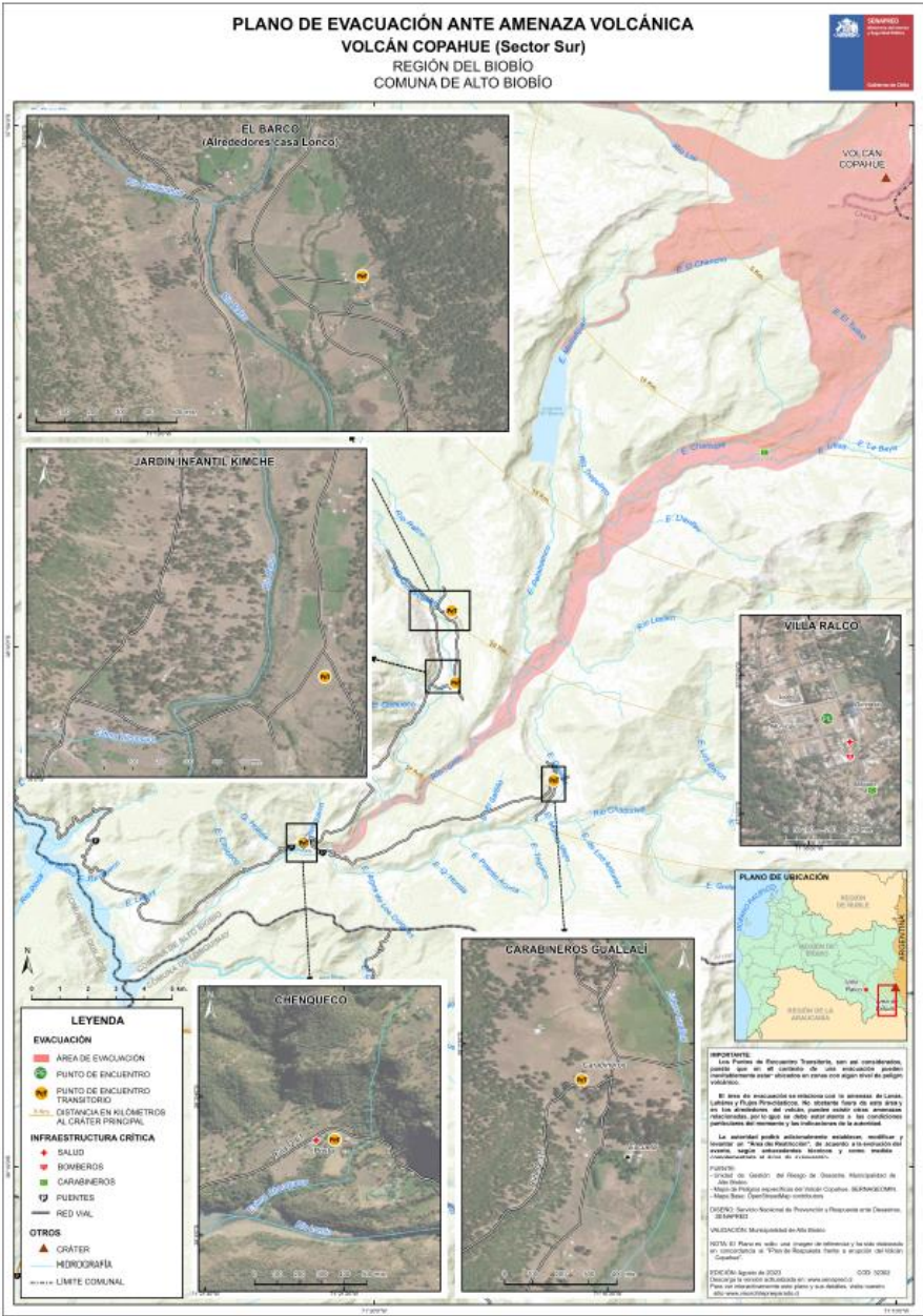
Figura 3. Plano de evacuación por amenaza del Volcán Copahue. (Sector Sur)
