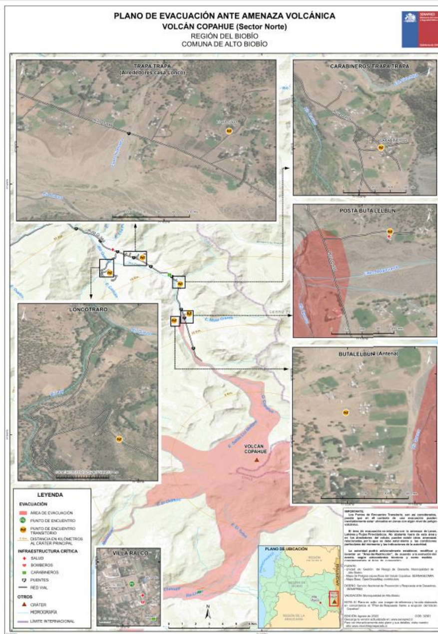
Figura 2. Plano de evacuación por amenaza del Volcán Copahue. (Sector Norte)
