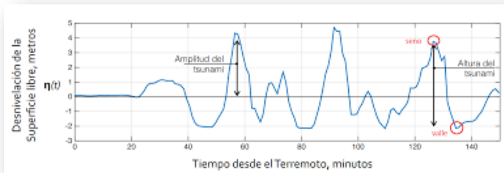
Figura 2: Definición de Parámetros de una onda de tsunami (mareógrafo de Coquimbo, 16 de septiembre de 2015). Fuente: Adaptación de Guía para la estimación de peligro de tsunami (2016).
