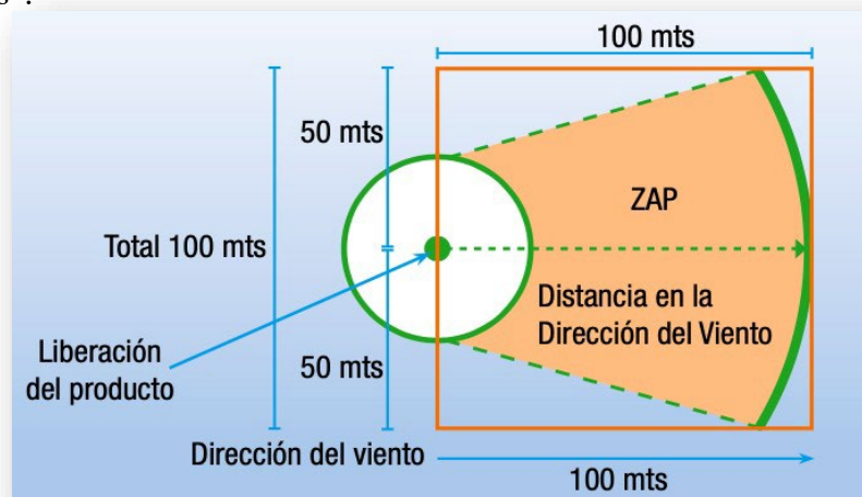
Figura 4: "Distancias de seguridad" Fuente, Academia Nacional de Bomberos, Guía de Instrucción Primera Respuesta, ante Incidentes con Materiales Peligrosos.
