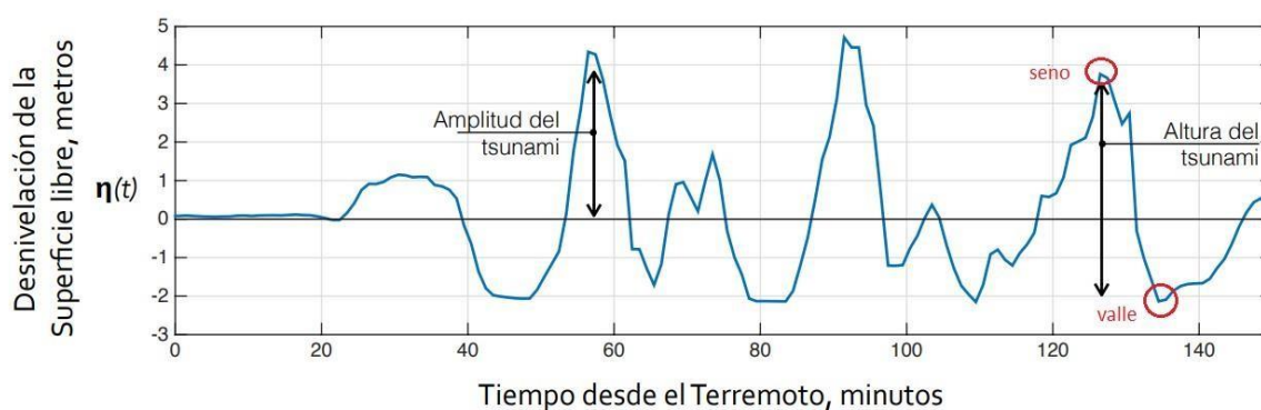
Figura 1 Definición de parámetros que definen una onda de tsunami (Mareógrafo de Coquimbo, 16 de septiembre de 2015). Fuente: Adaptación de Guía para la estimación de peligro de tsunami (2016).
