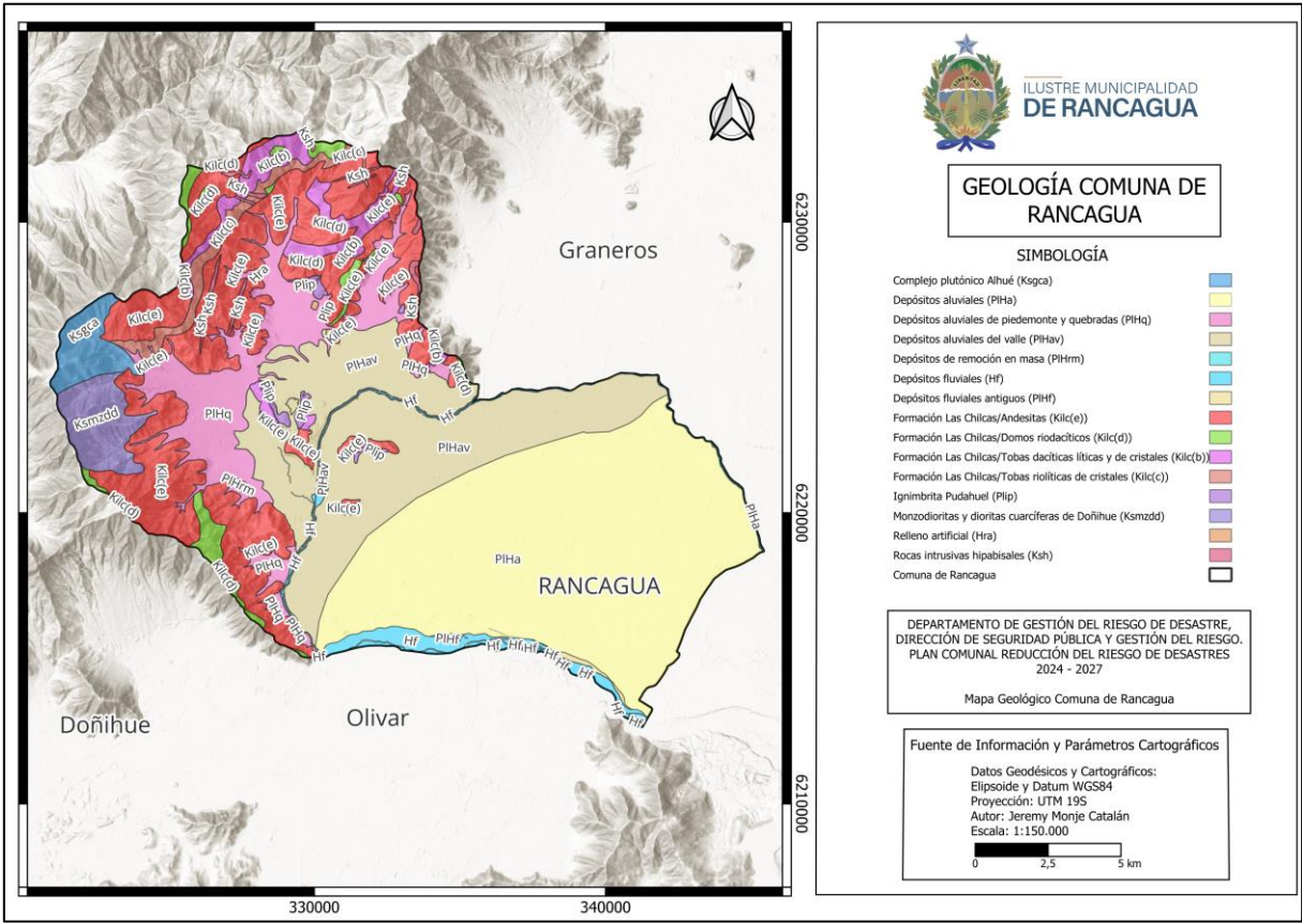
Figura 1. Mapa Geológico de la Comuna de Rancagua, modificado de la Carta Geológica Rancagua – San Vicente de Tagua Tagua, (2009).
