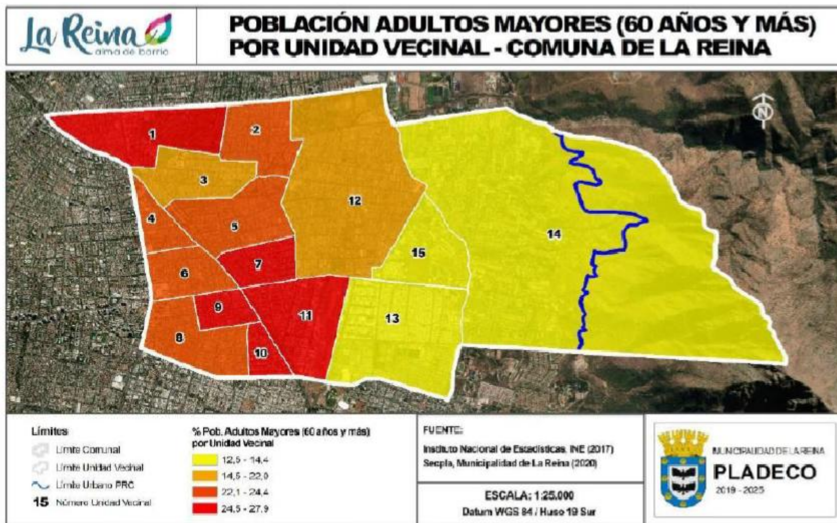
Figura N°2: Población de 60 años y más por unidad vecinal en la comuna de La Reina.
