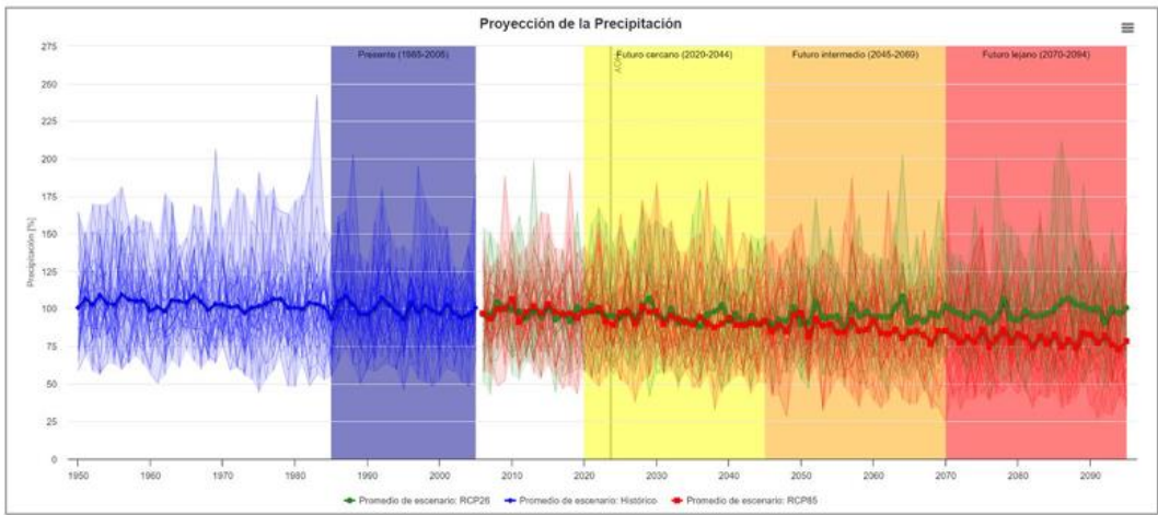
Gráfico 19 Proyección de precipitaciones, comuna de Linares
