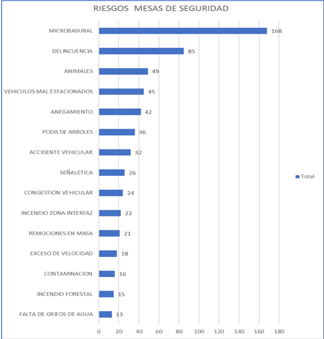
Gráfico 2: Tipos Riesgos
