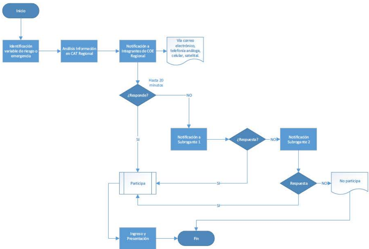
Diagrama de Flujo de Datos Nivel 1: Esquema general de la convocatoria.
